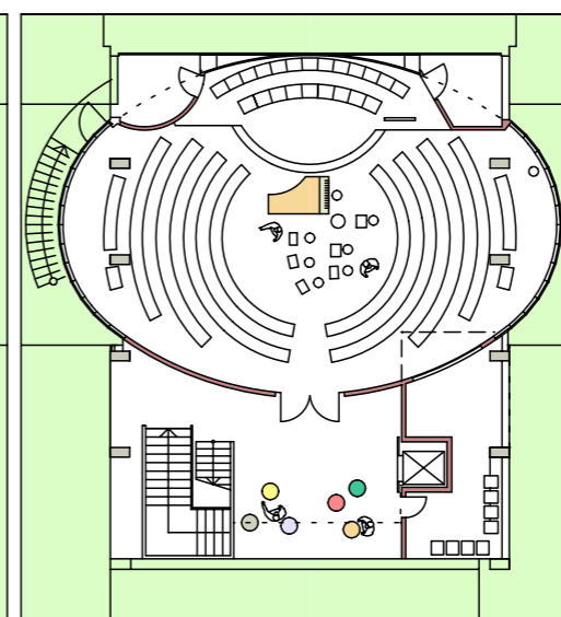
Konzert 115 Plätze
