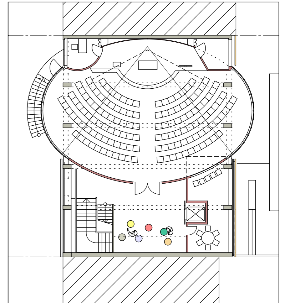
Grundriss Obergeschoß
