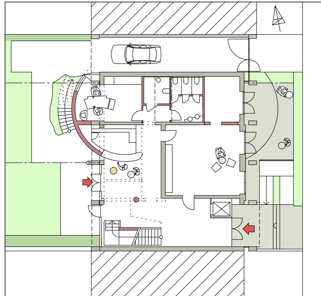
Grundriss Erdgeschoß
