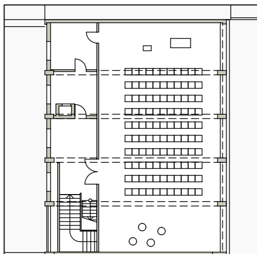
Grundriss OG Bestand
