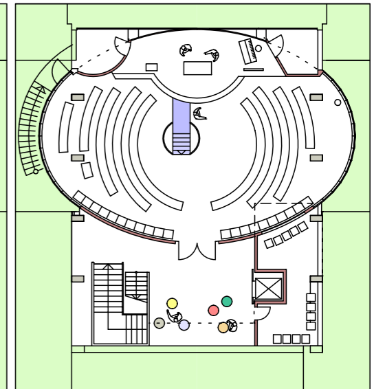
Taufgottesdienst 130 Plätze
