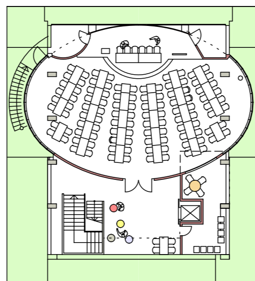
Konferenz 110 Plätze
