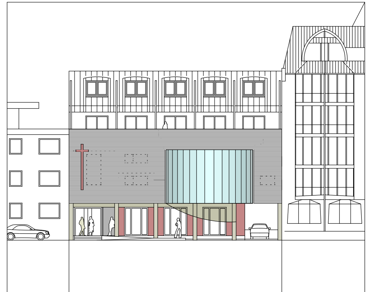
Ansicht Ost
